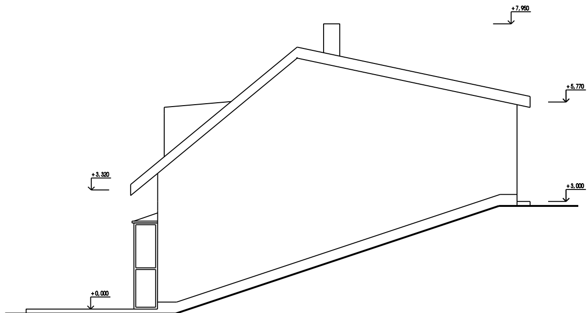
SEVERNÍ POHLED
