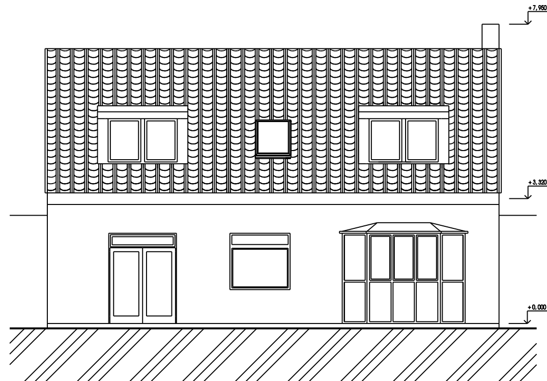
VÝCHODNÍ POHLED
