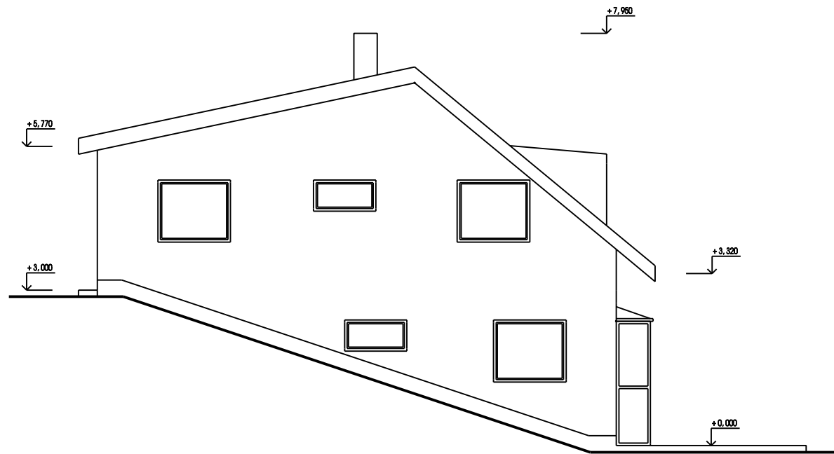
JIŽNÍ POHLED
